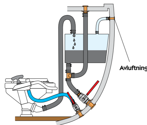
SEPTIKTANK ÖVER VATTENLINJEN
