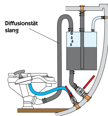
SEPTIKTANK ÖVER VATTENLINJEN
