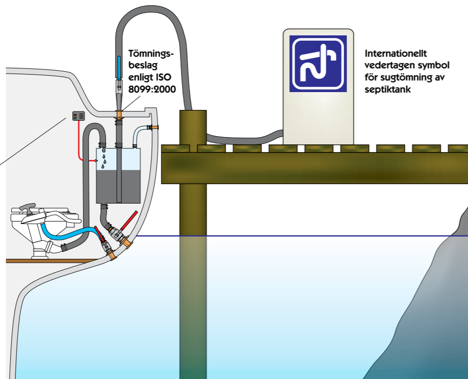
SEPTIKTANK ÖVER VATTENLINJEN
